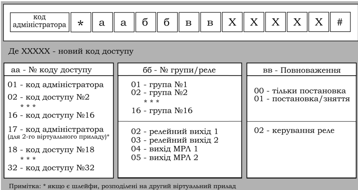
Рисунок 5 – Програмування кодів доступу
