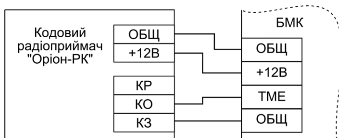
Рисунок 4 - Схема підключення кодового радіоприймача «Оріон-ПК»
