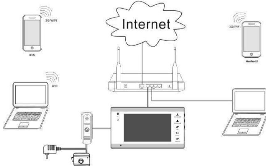
Рисунок 4-1. Проводное (LAN) подключение домофона к роутеру
