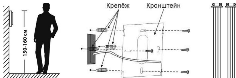
Рисунок 2. Высота установки, кронштейн, и разъемы подключения
