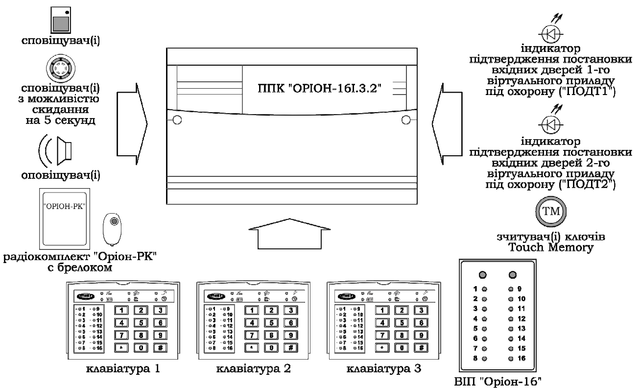
Рисунок 1 – загальний вигляд ППКО «Оріон 16І.3.2»
