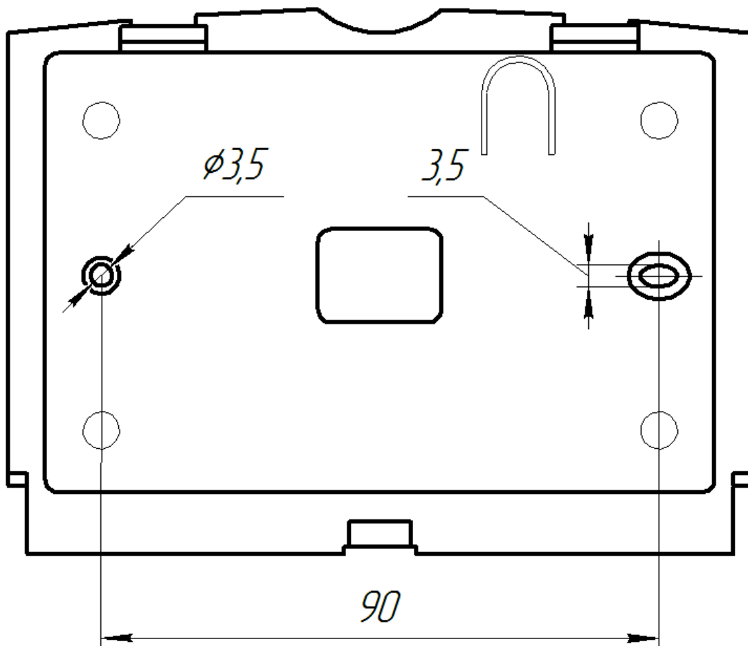
Рисунок 1 - Установочные размеры клавиатуры K-LED16
