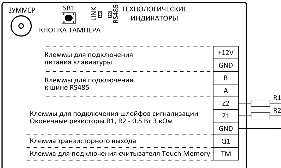
Рисунок 2 - Схема электрическая подключения
