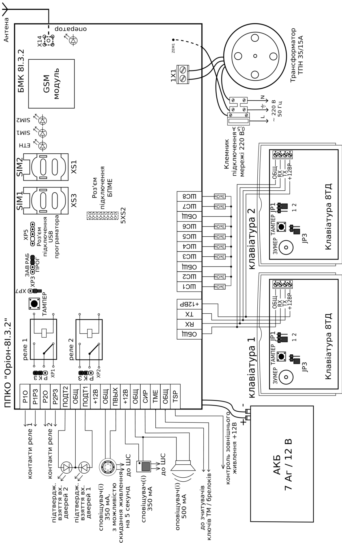
Рисунок А.2 – Схема підключення електрична ППКО «Оріон-8І.3.2»
